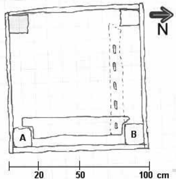
Grondplan waterput
