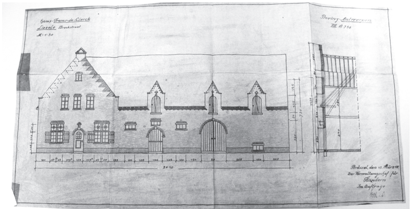
Het plan voor de hoeve van Frans De Clerck uit Liezele opgemaakt door Duitse architecten (©Algemeen Rijksarchief Brussel - Verwoeste gewesten)
