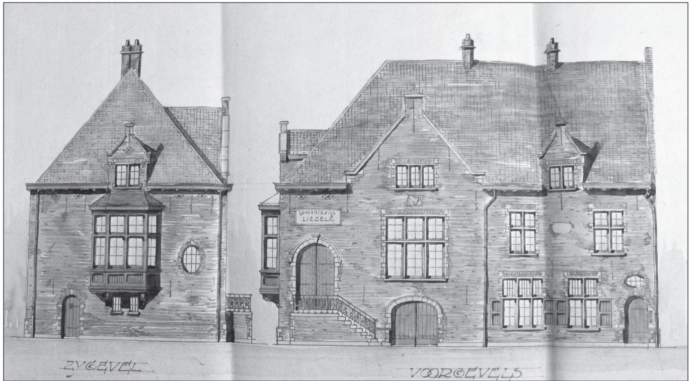
Plan van het gemeentehuis en de onderwijzerswoning (©Algemeen Rijksarchief Brussel)
