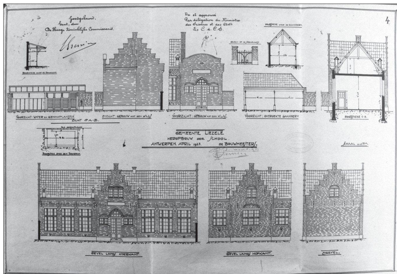
De plannen voor de nieuwe school uit 1923 (©Algemeen Rijksarchief Brussel - Verwoeste gewesten)
