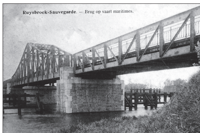
De spoorbrug te Ruisbroek werd toegankelijk gemaakt met balken en plankenvloer (Verzameling Georges Verbruggen)
