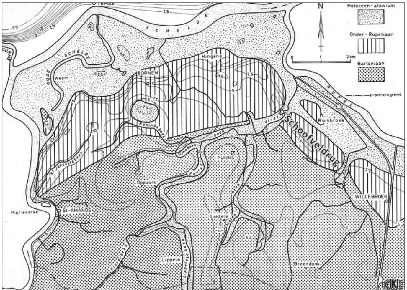
Afb. 8: De Schoofveldrug weergegeven op de geologische kaart van Klein-Brabant.
